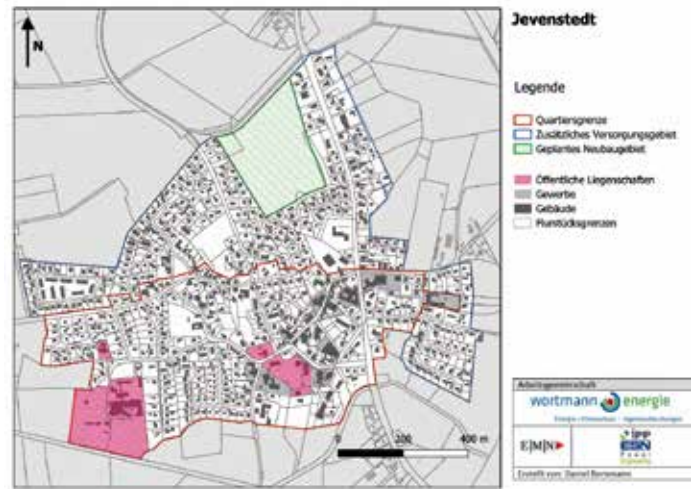
Abbildung 2: Geplantes Ausbaugelände des Wärmenetzes.
